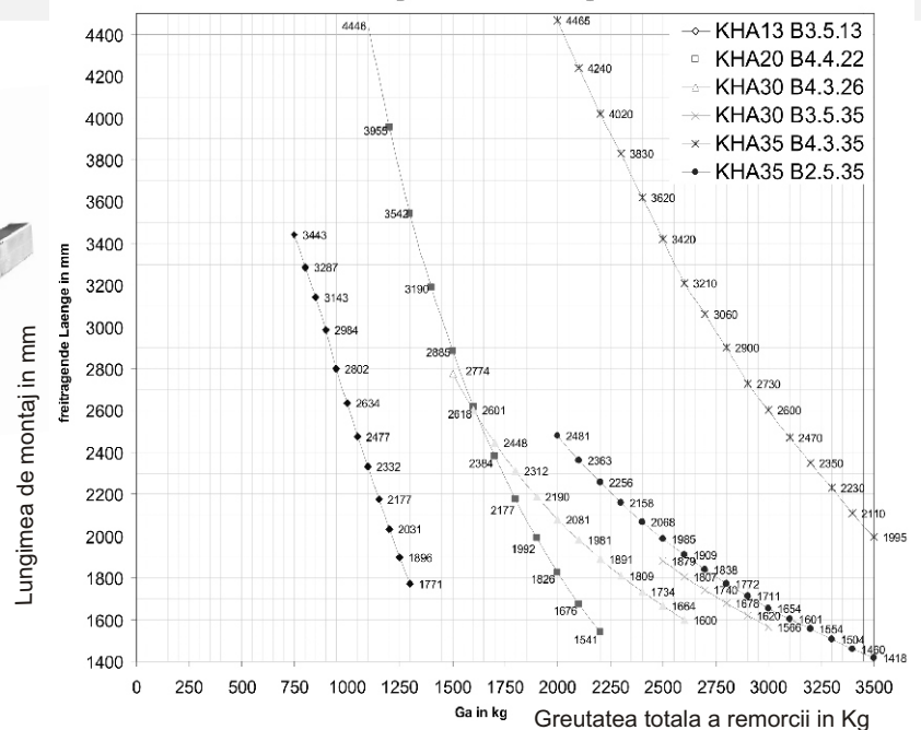
Alegerea lungimii barei KHA freitragende Deichsellaenge KHA
